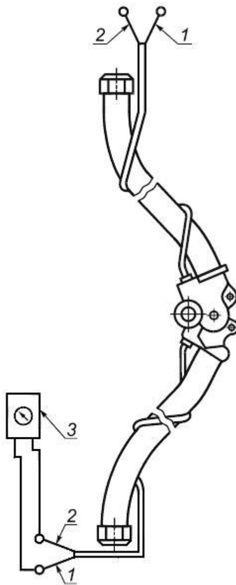
1, 2 - жила кабеля; 3 - мегомметр
