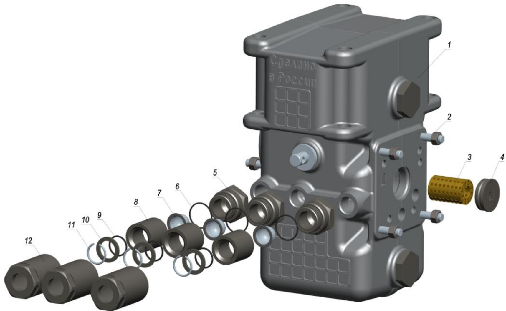
1 - камера, 2 - гайка, 3 - фильтр, 4 - пробка, 5 - штуцер, 6 - кольцо, 7 - фильтр, 8 - ниппель, 9 - кольцо, 10 - шайба, 11 - кольцо, 12 - гайка.
