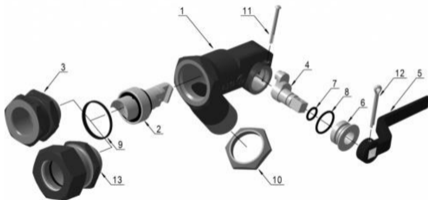
Кран концевой 4314Б
