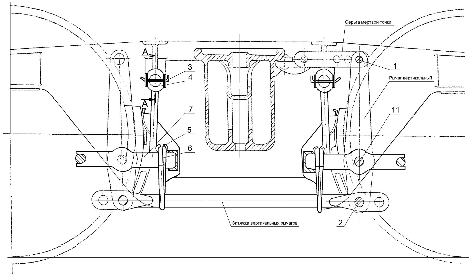
Б вариант Предохранитель валика подвески тормозного башмака (ОАО «РИТМ»)
