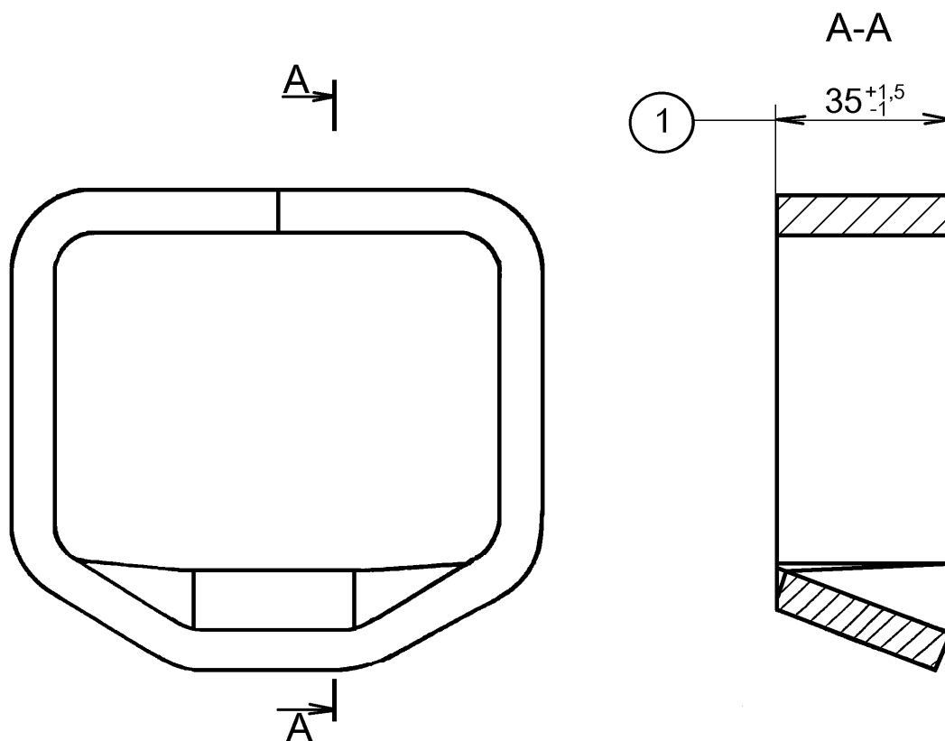
Рисунок 5 – Закладка триангеля 100.40.008-2
