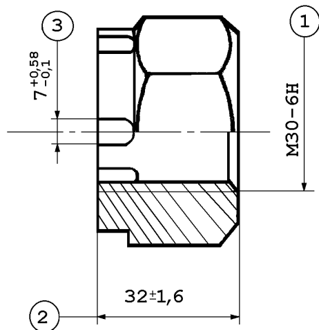
Рисунок 10 – Гайка 100.40.012-1
