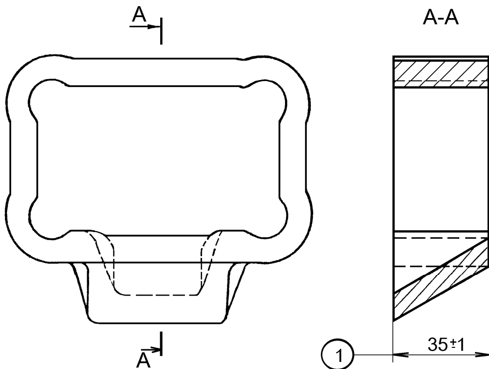
Рисунок 5 – Закладка триангеля 100.40.008-2
