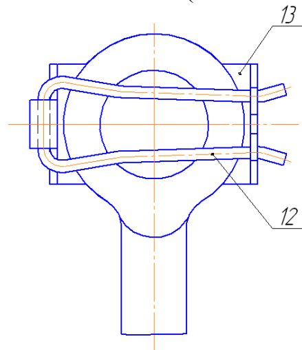
Б вариант Предохранитель валика подвески тормозного башмака (ОАО «РИТМ»)
