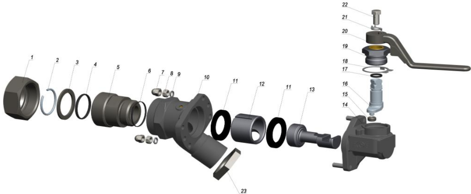
1 - гайка, 2 - кольцо, 3 - шайба, 4 - кольцо, 5 - штуцер, 6 - кольцо, 7 - гайка, 8 - гайка, 9 - шайба, 10 - колено, 11 - воротник, 12 - распорка, 13 - клапан, 14 - корпус, 15 - втулка, 16 - кривошип, 17 - кольцо, 18 - шайба, 19 - опора, 20 - ручка, 21 - шайба, 22 - болт, 23 - контргайка.
